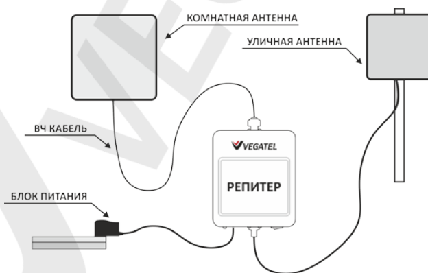
Пример схемы подключения репитера
